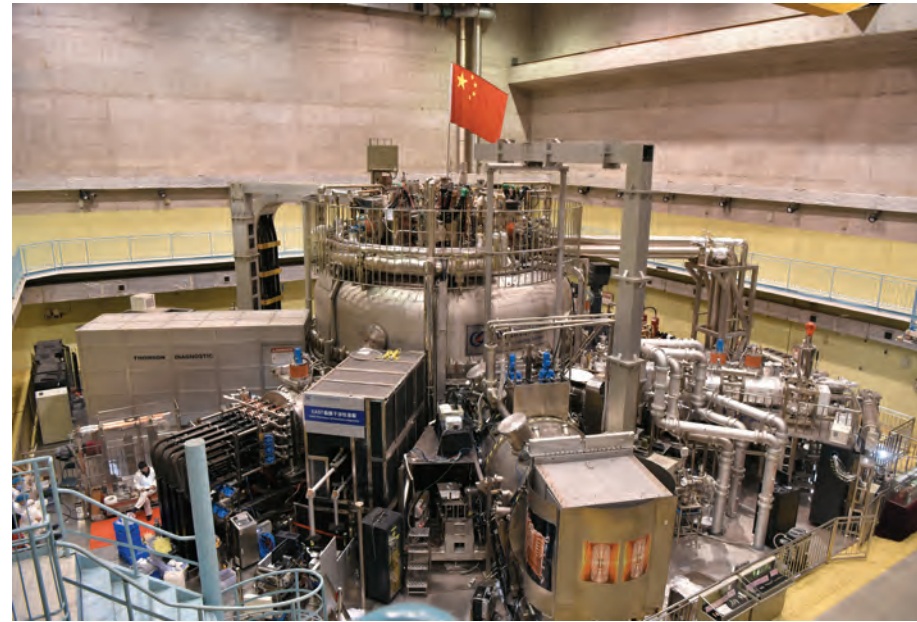
“人造小太阳”全超导托卡马克核聚变实验装置
